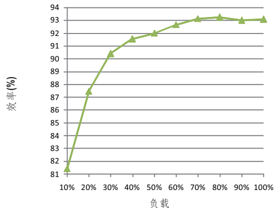
◎ 以上曲线是在230VAC下测
